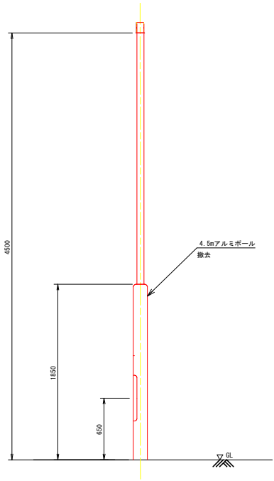
照明柱詳細図 S=1:20
